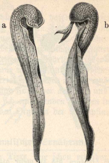
Abb. 27. Krug a. von Sarracenia , b. von Darlingtonia .
