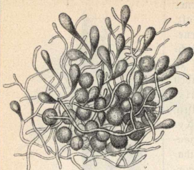
Abb. 35. Kohlrabihäuschen einer Ameisen-Pilzkultur.
