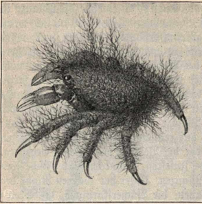
Abb. 32. Spitzkrabbe (Hyas) mit Algenbesatz.
