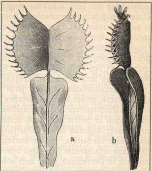
Abb. 30. Blatt der Venusfliegenfalle. a. geöffnet, b. geschlossen.
