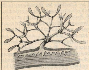
Abb. 17. Mistel, in einem Baumzweige wurzelnd.
