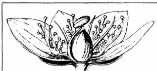
Abb. 59. Blüte vom Studentenröschen; der letzte Staubbeutel überdeckt die Narbe.
