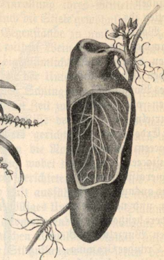
Abb. 15. Dischidia Rafflesiana mit Blattkrügen.
