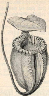
Abb. 26. Ranne von Nepenthes .
